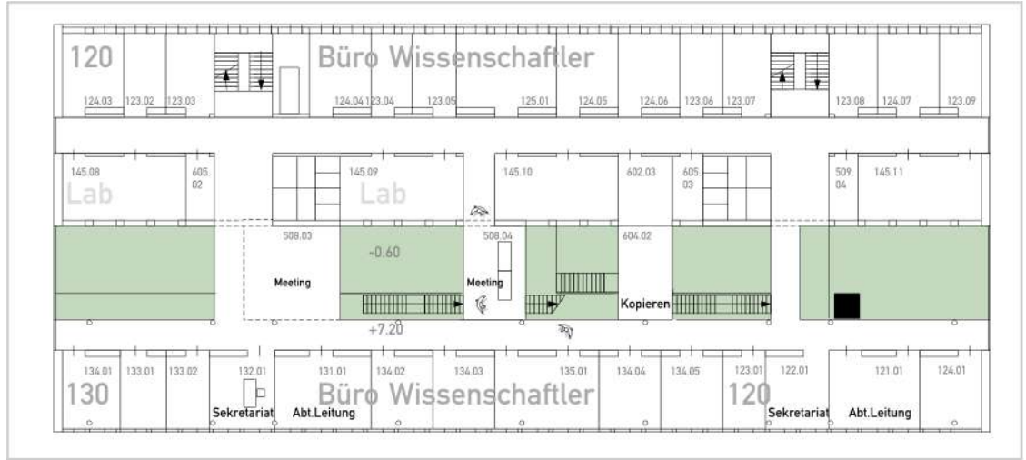
^^ Grundriss 2.0G
