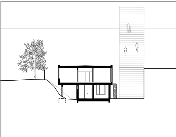
Schnitt
